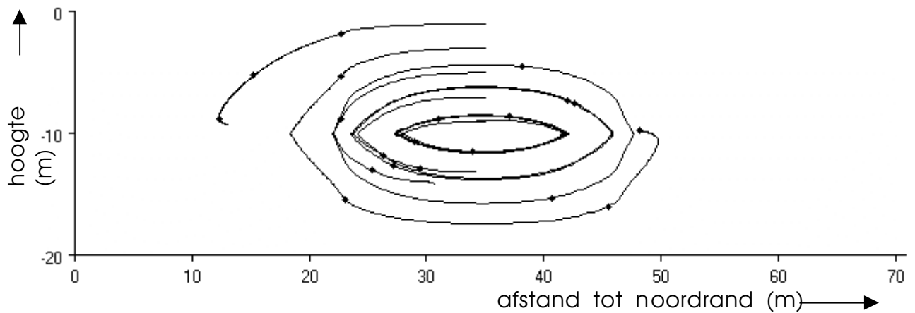
Figuur 3: De vijf spiraalvormige stroombanen (figuur 2), geprojecteerd op een noord-zuid doorsnede.
