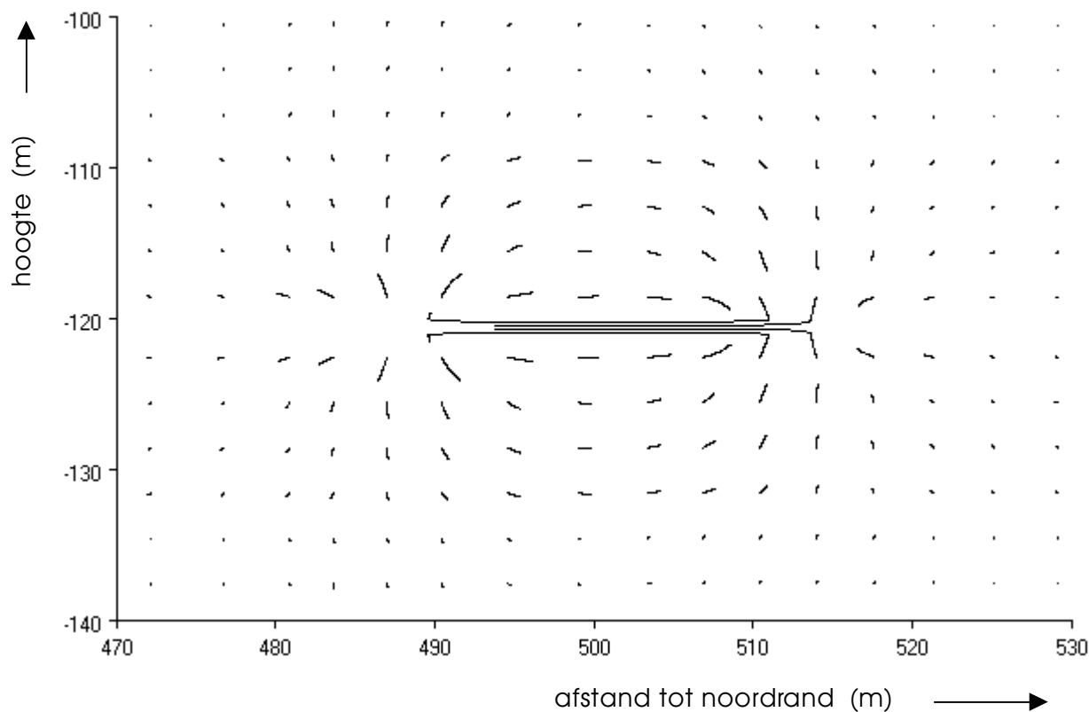
Figuur 5: Asymmetrische wervels boven en onder een (1 m) dunne anisotrope laag.
