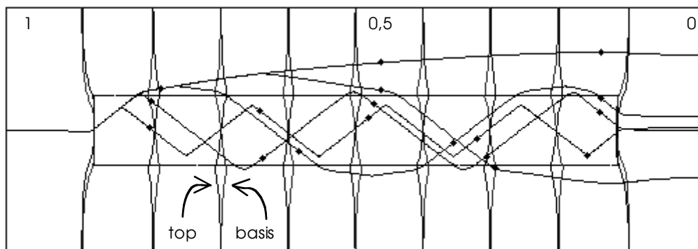
Figuur 2: Bovenaanzicht van het twee-lagen testmodel met isohypsen in beide lagen en vijf stroombanen.
